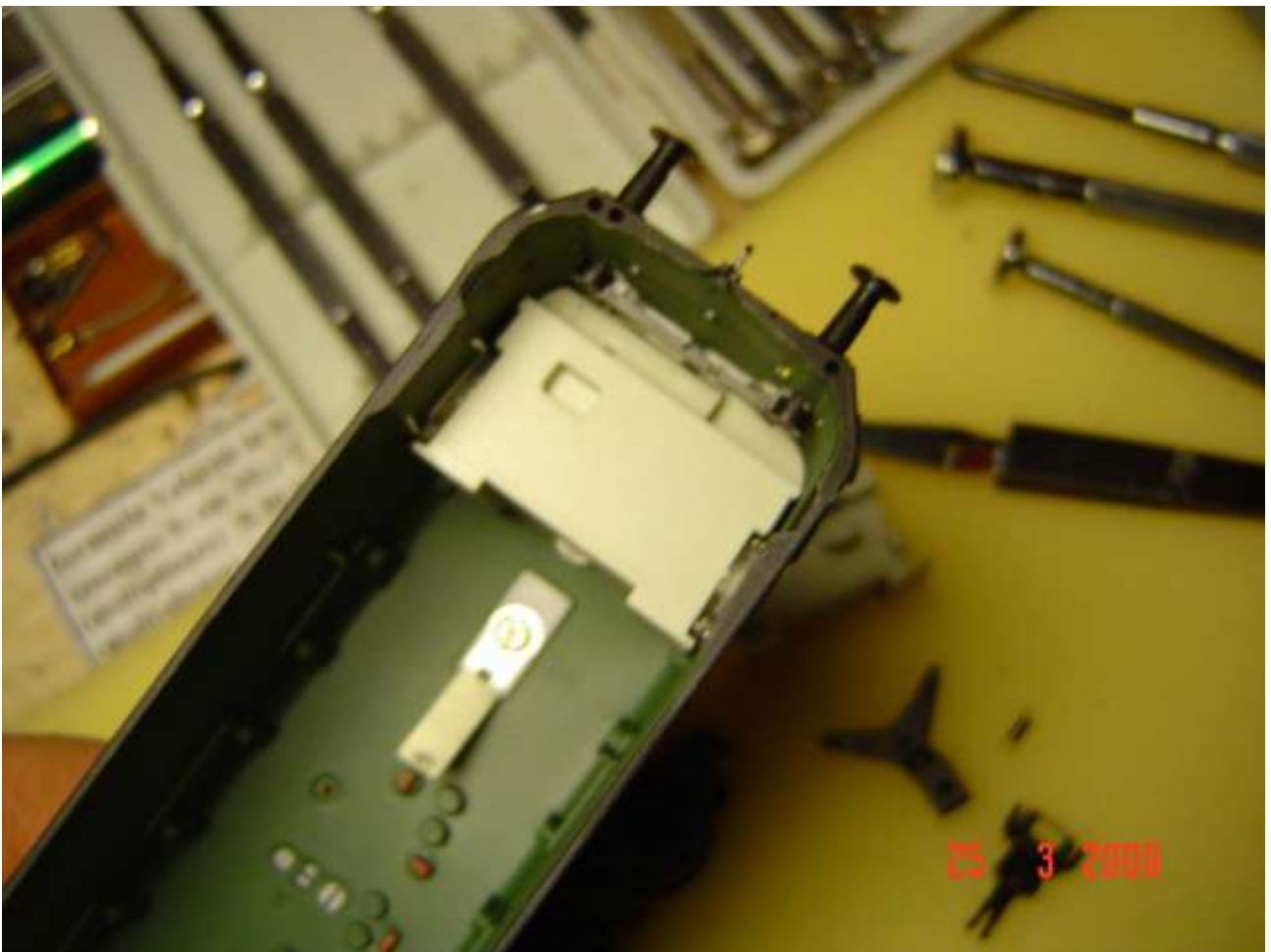
Foto n. 25: particolare dei fori sul bordo della carrozzeria dell' E 41 DB Märklin
