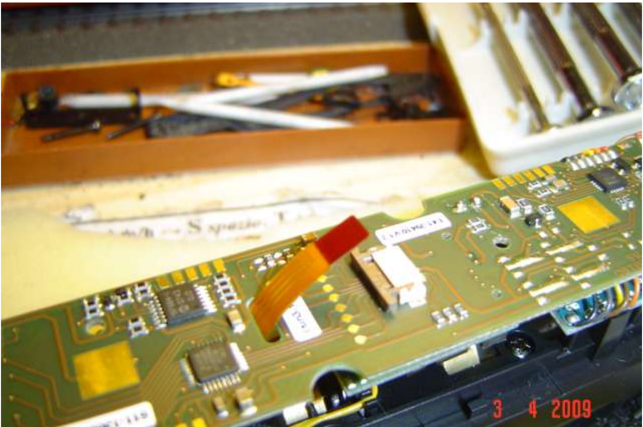
Foto B: la piattina di collegamento (stesso principio delle Sim Card dei telefoni cellulari) da staccare dal connettore (qui si vede aperto, al centro esatto, operazione necessaria per sollevare il circuito stampato nella E 41
