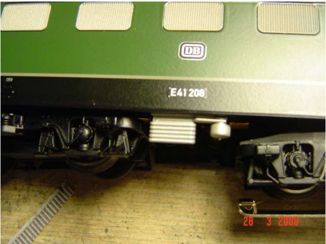
Foto n. 16: la E 41 DB, particolare delle griglie e della serpentina nel sottocassa
