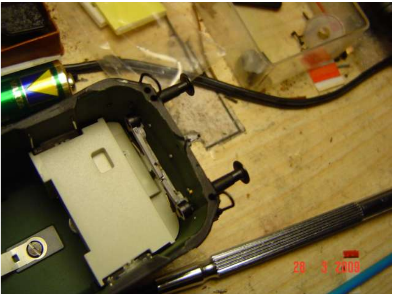
Foto n. 26: in quei fori vanno inseriti i tubi dei rec dell' E 41 DB Märklin
