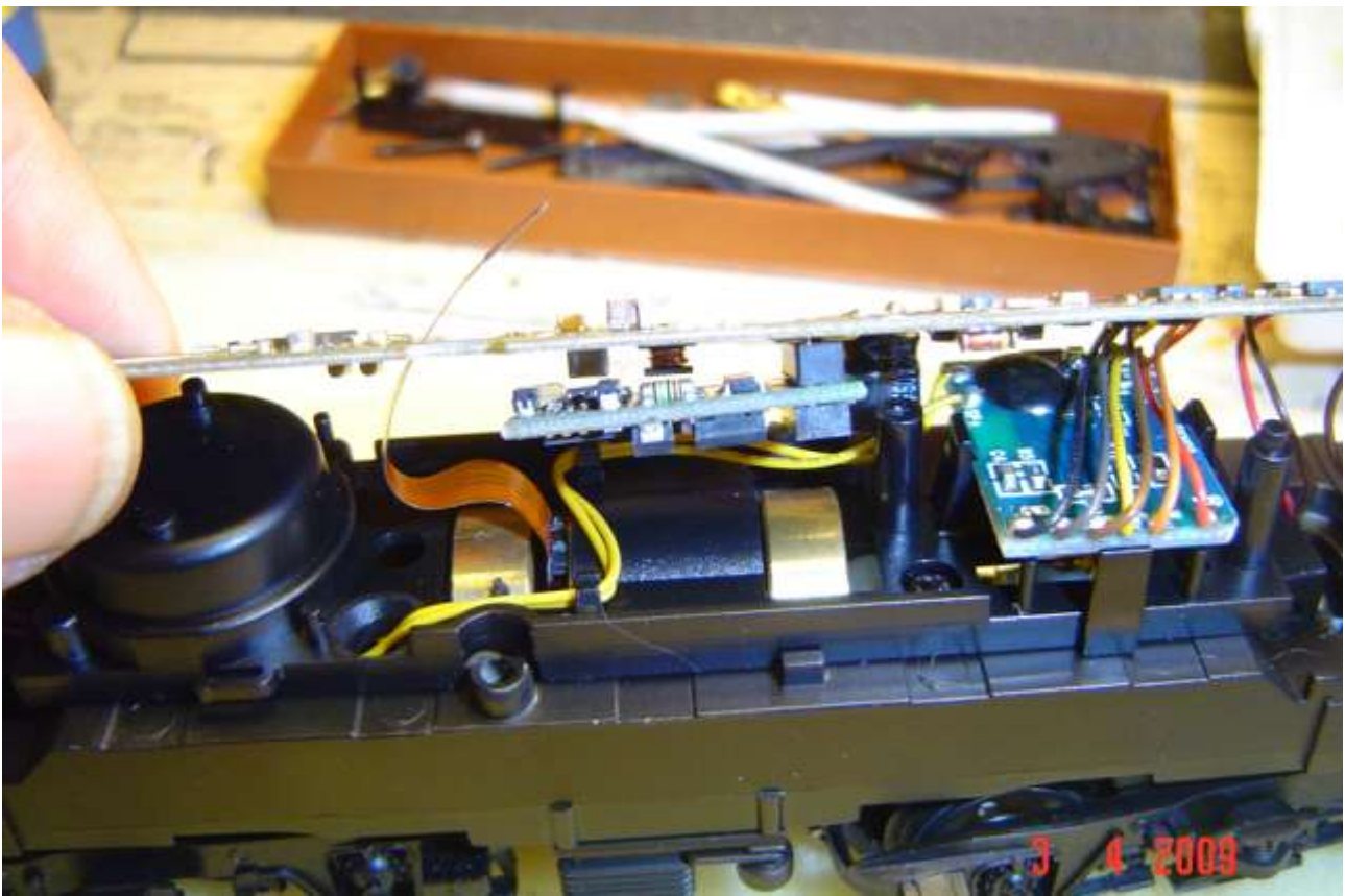
Foto C: il circuito stampato è solo appoggiato all'altoparlante a sinistra, notate la seconda vite da svitare in basso subito a sinistra del circuito elettronico più piccolo a destra nella foto.
