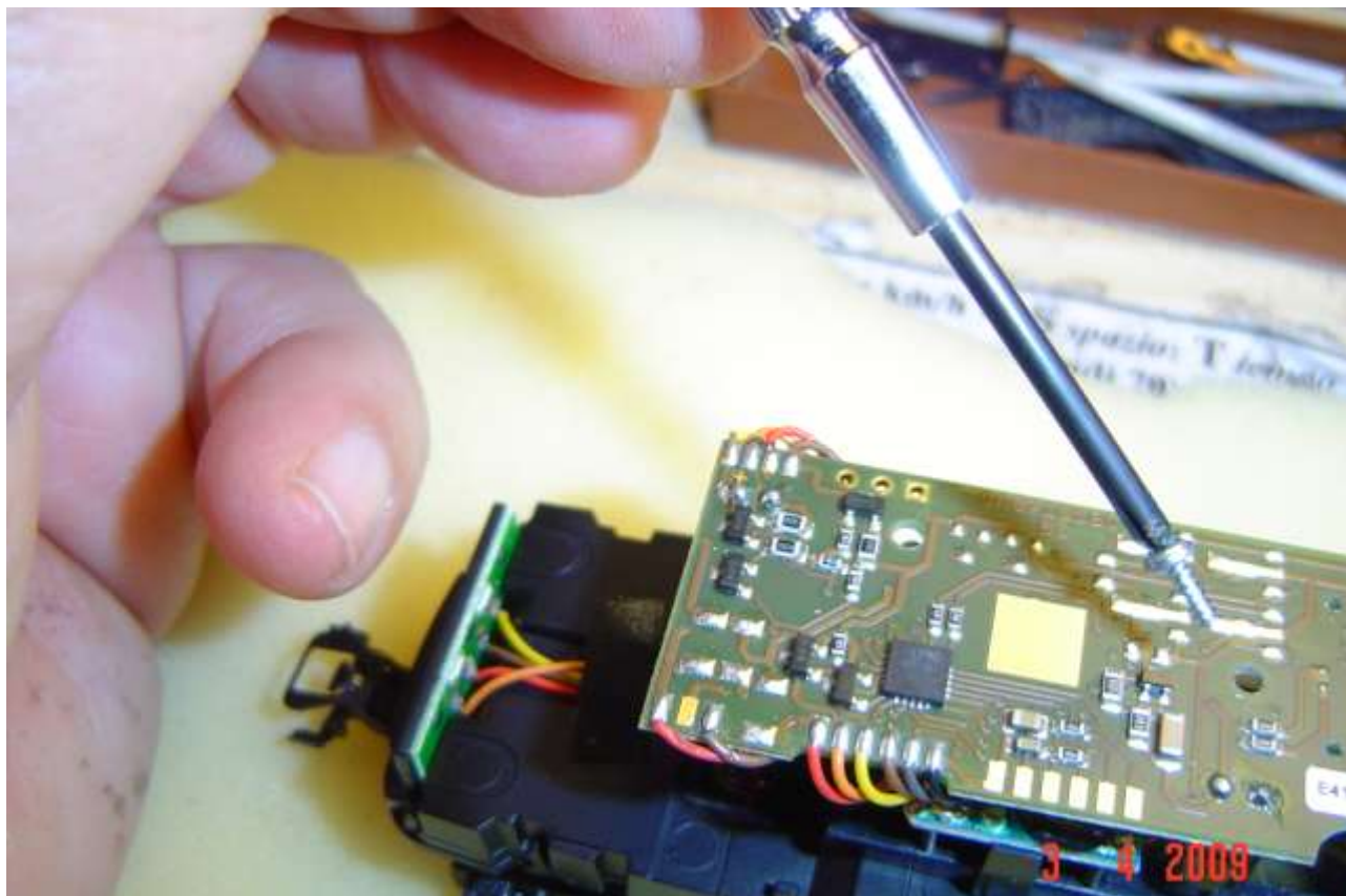
Foto A: la prima vite da allontanare per sollevare il circuito stampato nella E 41
