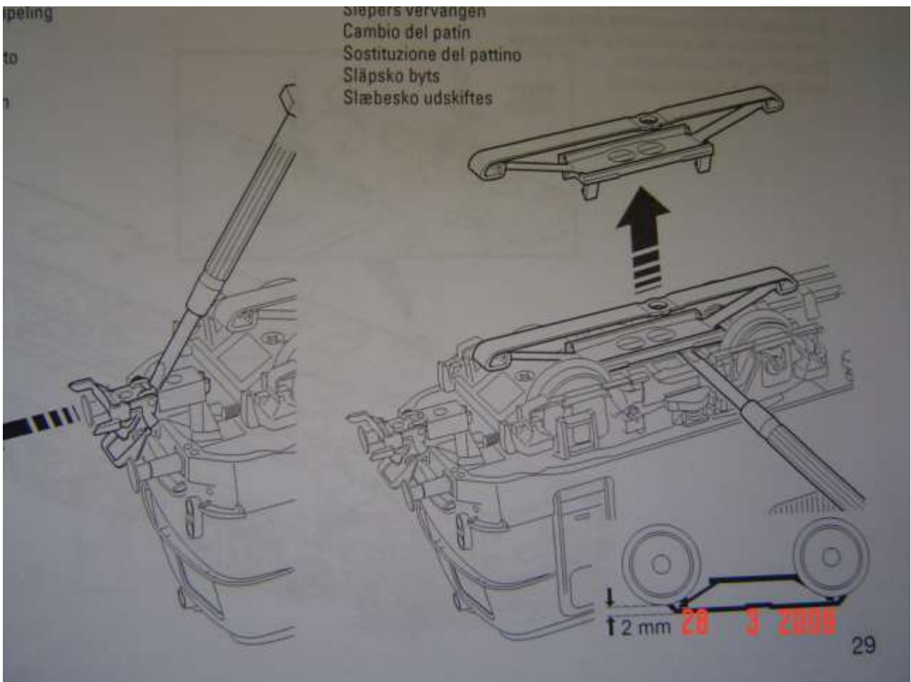
Foto n. 21: le istruzioni per allontanare gancio e pattino nella E 41 DB
